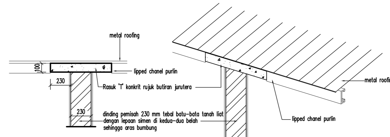
BUTIRAN 'B' DINDING PEMISAH 'T' SCALE : 1 : 25
