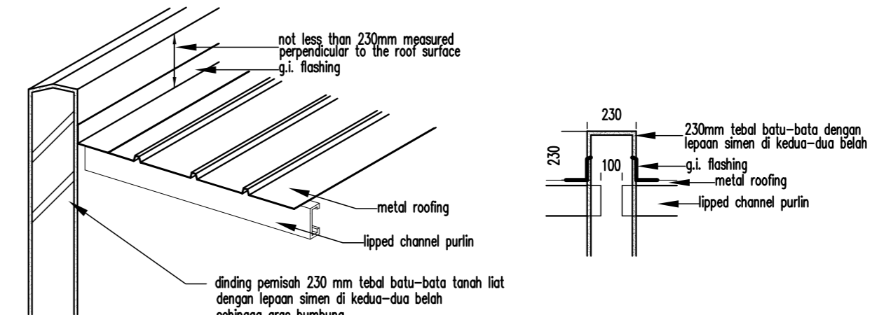
BUTIRAN 'A' PERINCIAN DINDING PEMISAH SCALE : 1 : 25
